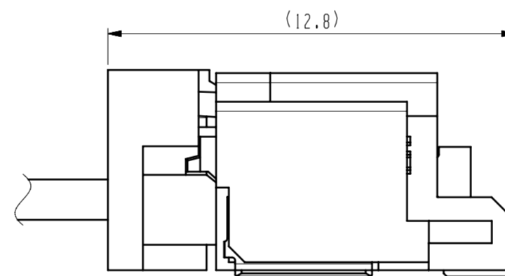
与护套配合后尺寸
